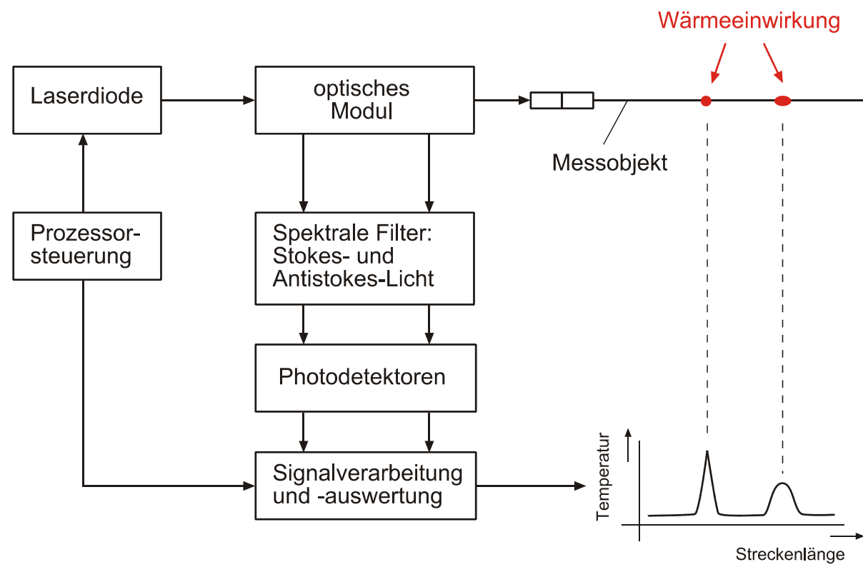
Bild 4.2: Prinzip der orts aufgelösten Temperaturmessung (Quelle: LIOS)
